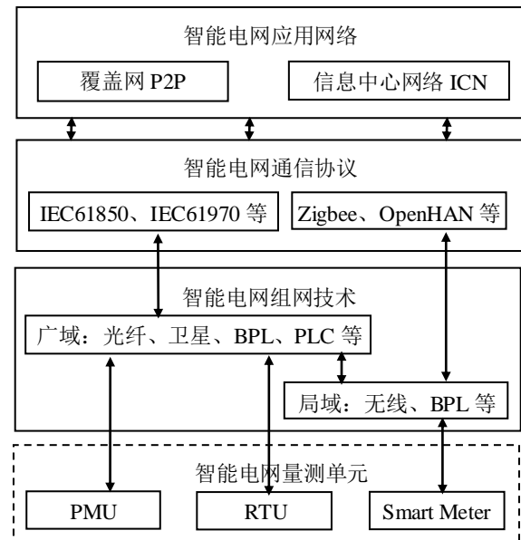
图 3 智能电网通信网络系统
