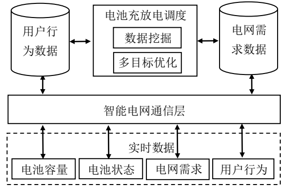
图 9 V2G 系统构架图
