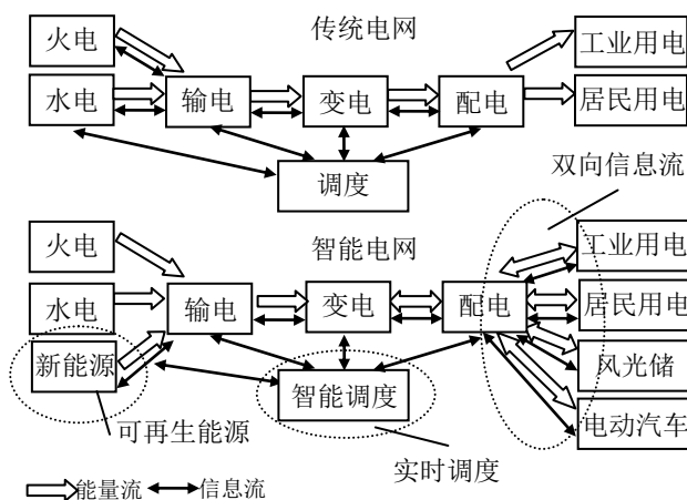
图1 传统电网和智能电网区别示意图
