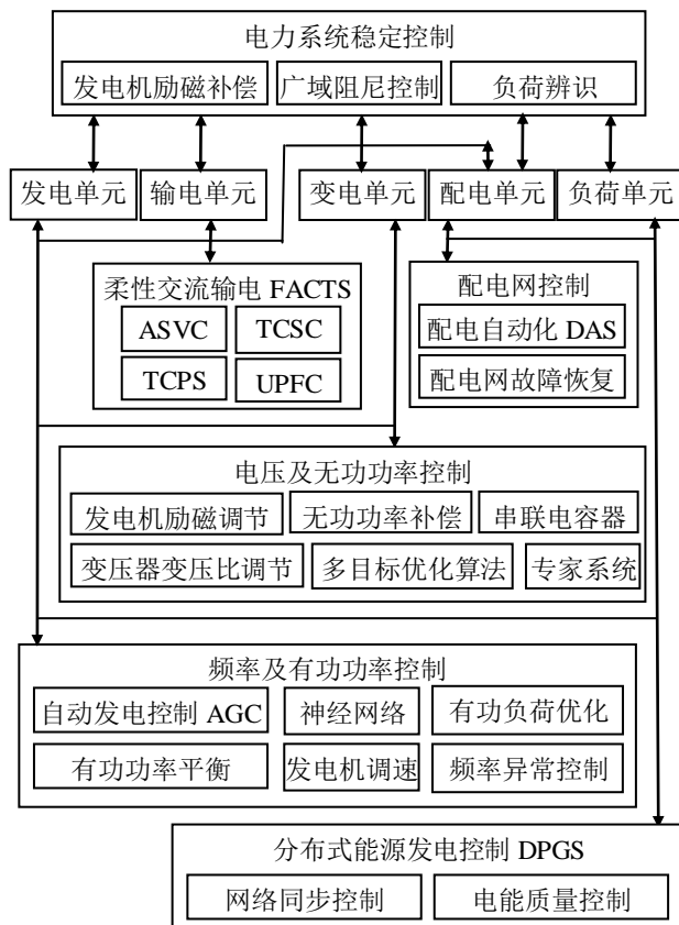
图7 智能控制执行系统
