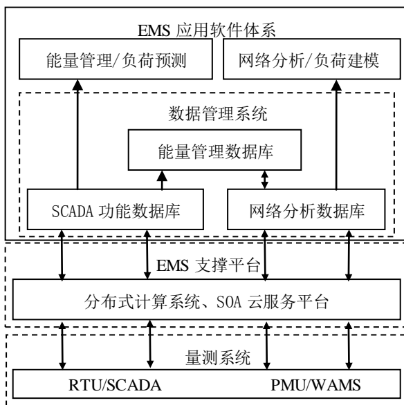
图 11 智能电网规划调度系统体系构架
