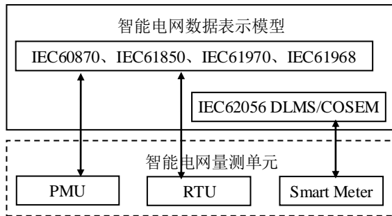
图5 智能电网数据表示模型
