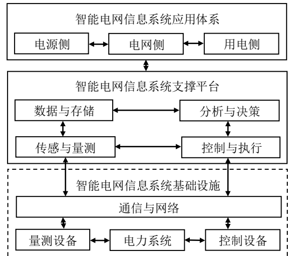
图 2 智能电网信息系统体系结构示意图
