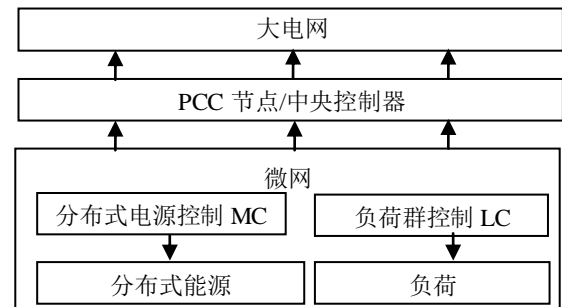
图 13 微网结构图
