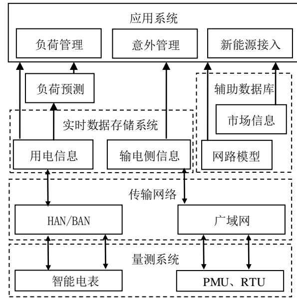
图 12 智能电网需求侧响应系统
