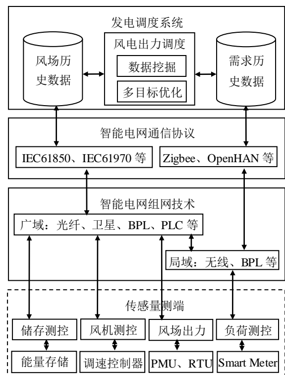
图 8 智能电网分析决策系统
